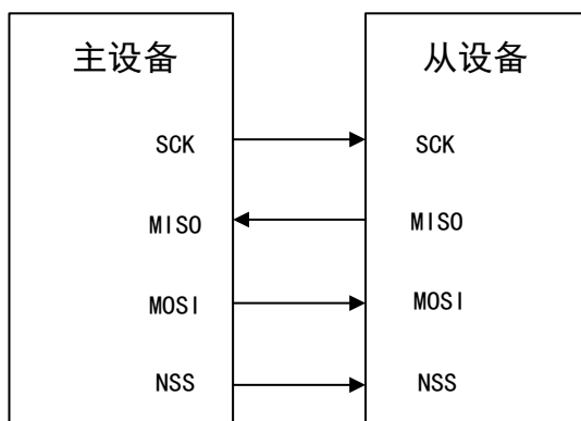
图 110 半双工模式连接
