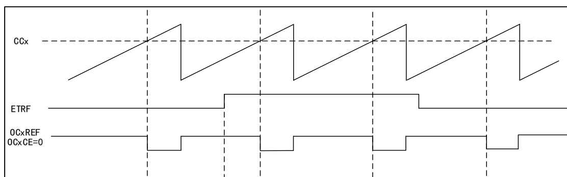
图 39 OCxREF 时序图
