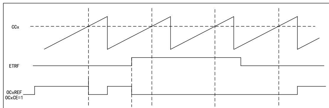
图 40 OCxREF 时序图
