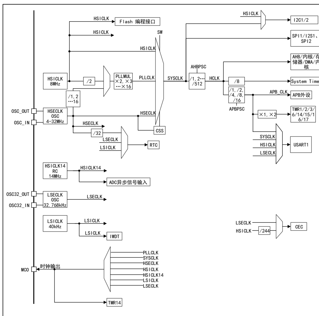
图 4APM32F051x6x8 时钟树
